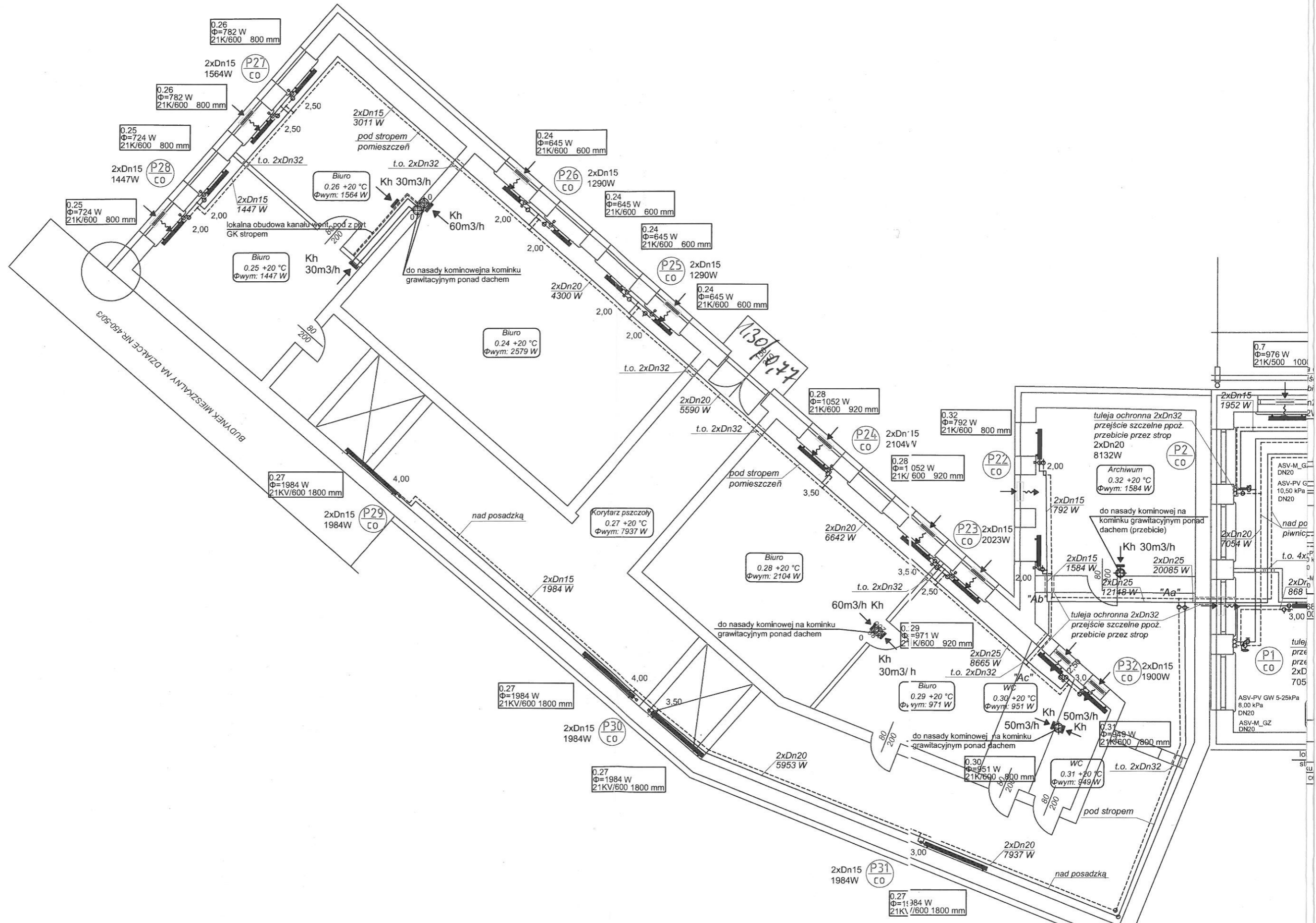
BUDYNEK PARTEROWY
