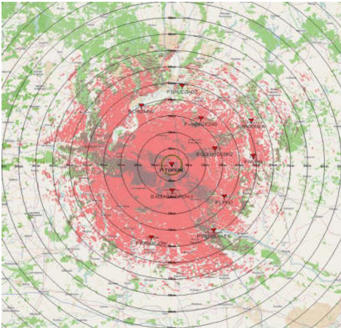
Rys. 23 przedstawia zasięgi teoretyczne przemiennika głównego dla stacji mobilnych
