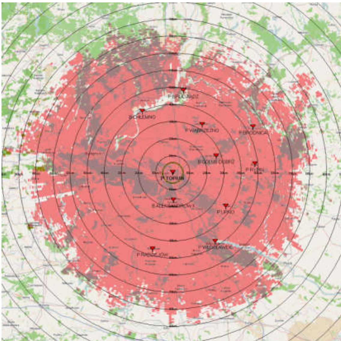
Rys. 24 przedstawia zasięgi nadajnika głównego w relacjach stacji bazowych wyniesionych
